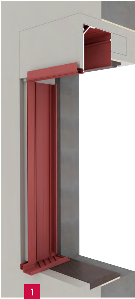
Montage der gedämmten Blindstockzarge mit Beschattungskasten und wasserführender Ebene im Rohbau
